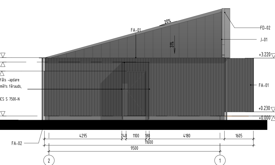
FASĀDE ASĪS 2- 1 M 1:100
