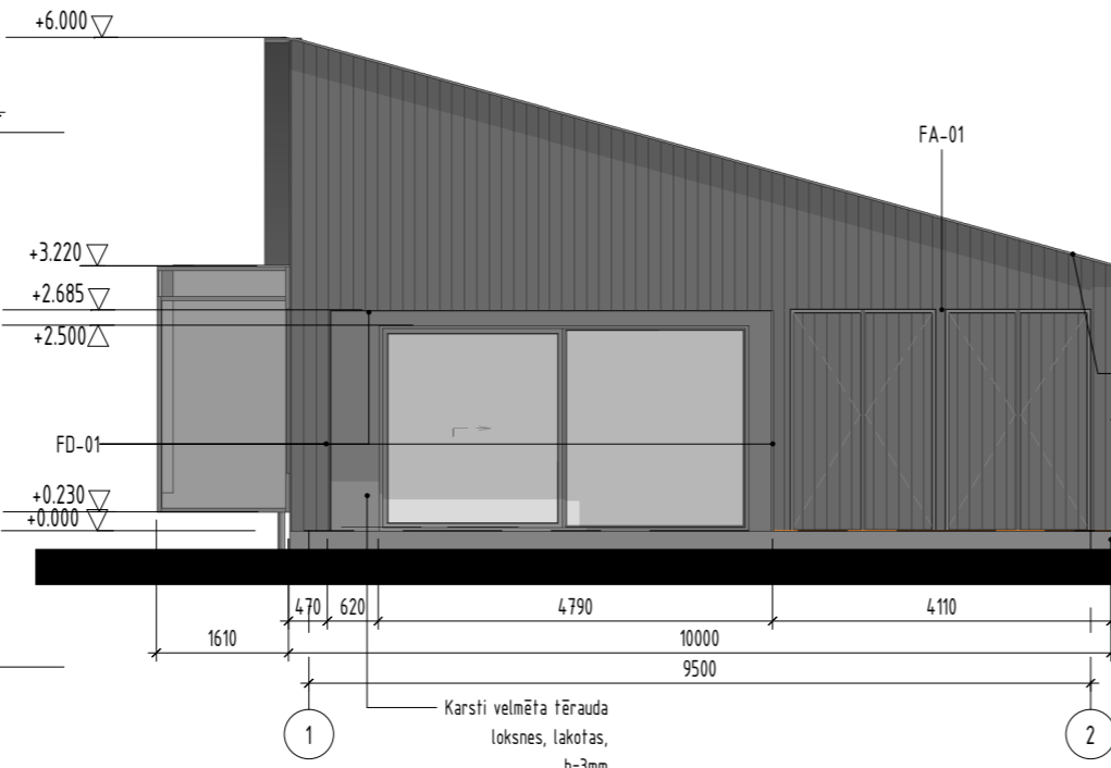
FASĀDE ASĪS 1- 2 M 1:100
