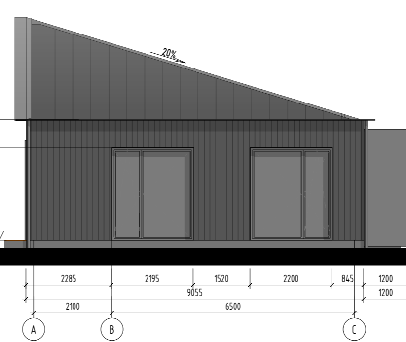
FASĀDE ASĪS A- C M 1:100
