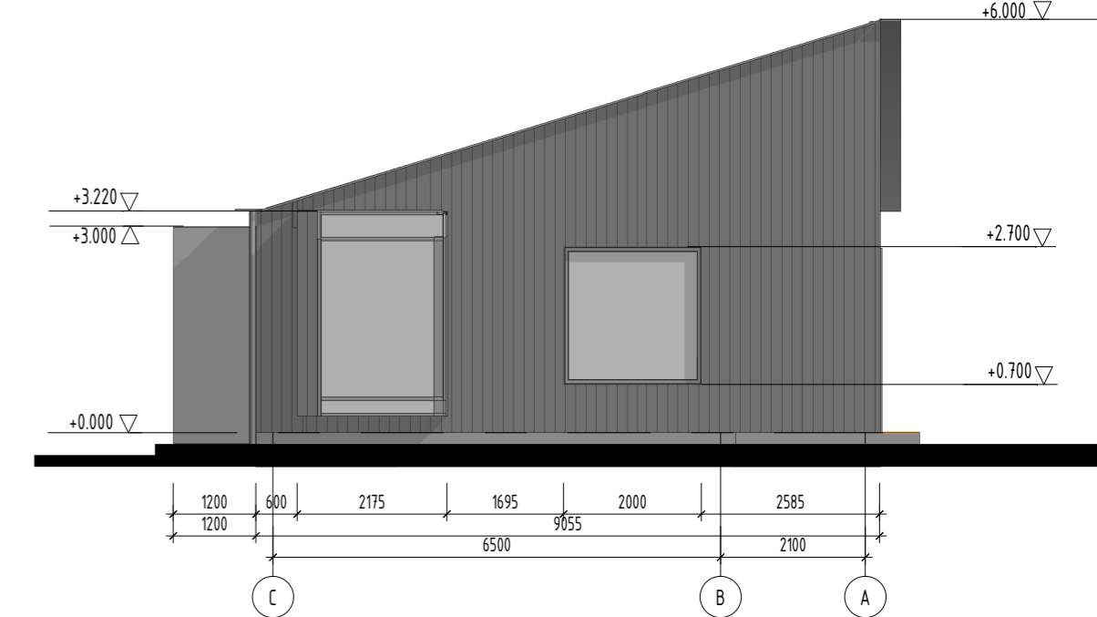
FASĀDE ASĪS C- A M 1:100
