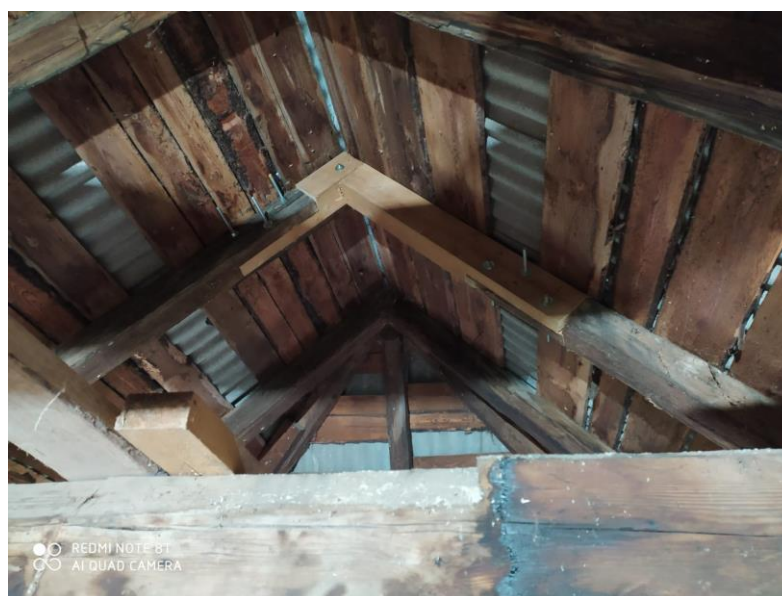
3. attēls – Asīs 2/7-A/C veikta jumta saišķu protezēšana un jumta spāru protezēšana.
